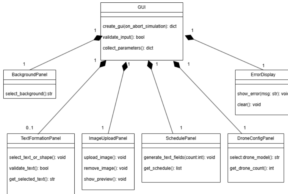
Abbildung 5.1: Klassendiagramm für Komponente \langle C10 \rangle
