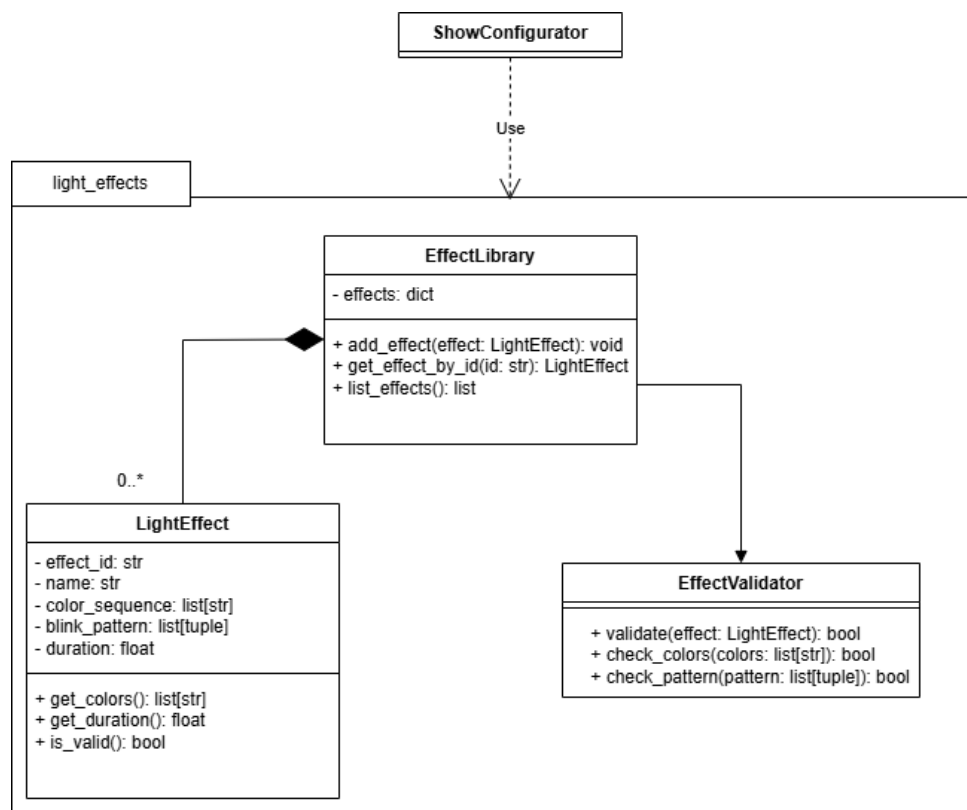
Abbildung 5.5: Klassendiagramm für Komponente \langle C40 \rangle
