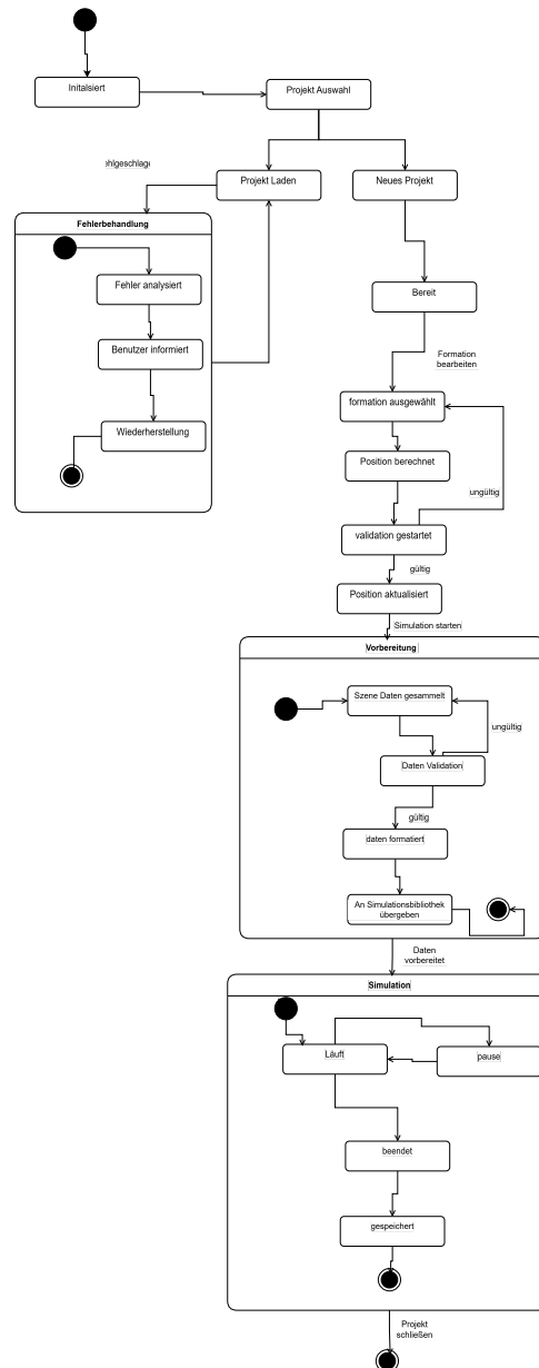
Abbildung 3.4: Zustandsdiagramm: Projektmanagment-Modul
