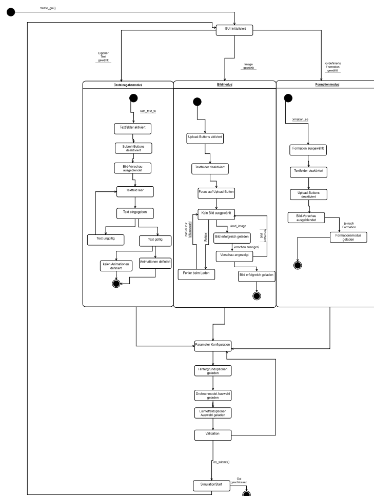
Abbildung 3.2: Zustandsdiagramm: GUI
