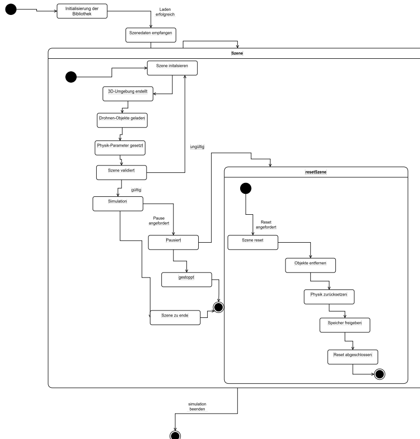
Abbildung 3.5: Zustandsdiagramm: Simulationsbibliothek
